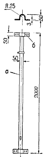
Рис. 27. Стойки переносные для установки сетки
